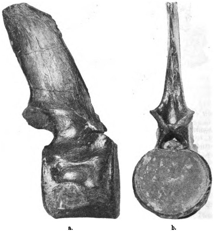
Fig. 4. Plesiosaurus limnophilus KOKEN. Der Halswirbel. \frac{2}{3} nat. Gr.
